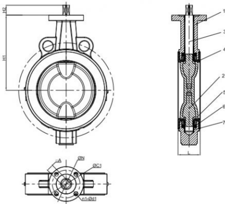
Bản vẽ kỹ thuật van bướm gang đĩa inox tay gạt
