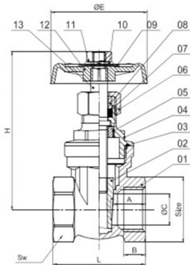
Bản vẽ kỹ thuật van cửa đồng
